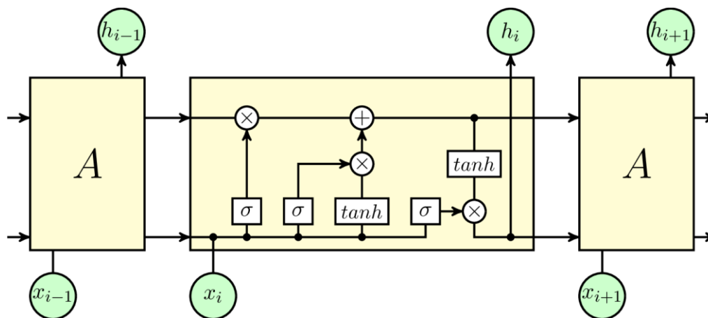
Рис. 3. Структура рекуррентной нейронной сети LSTM
